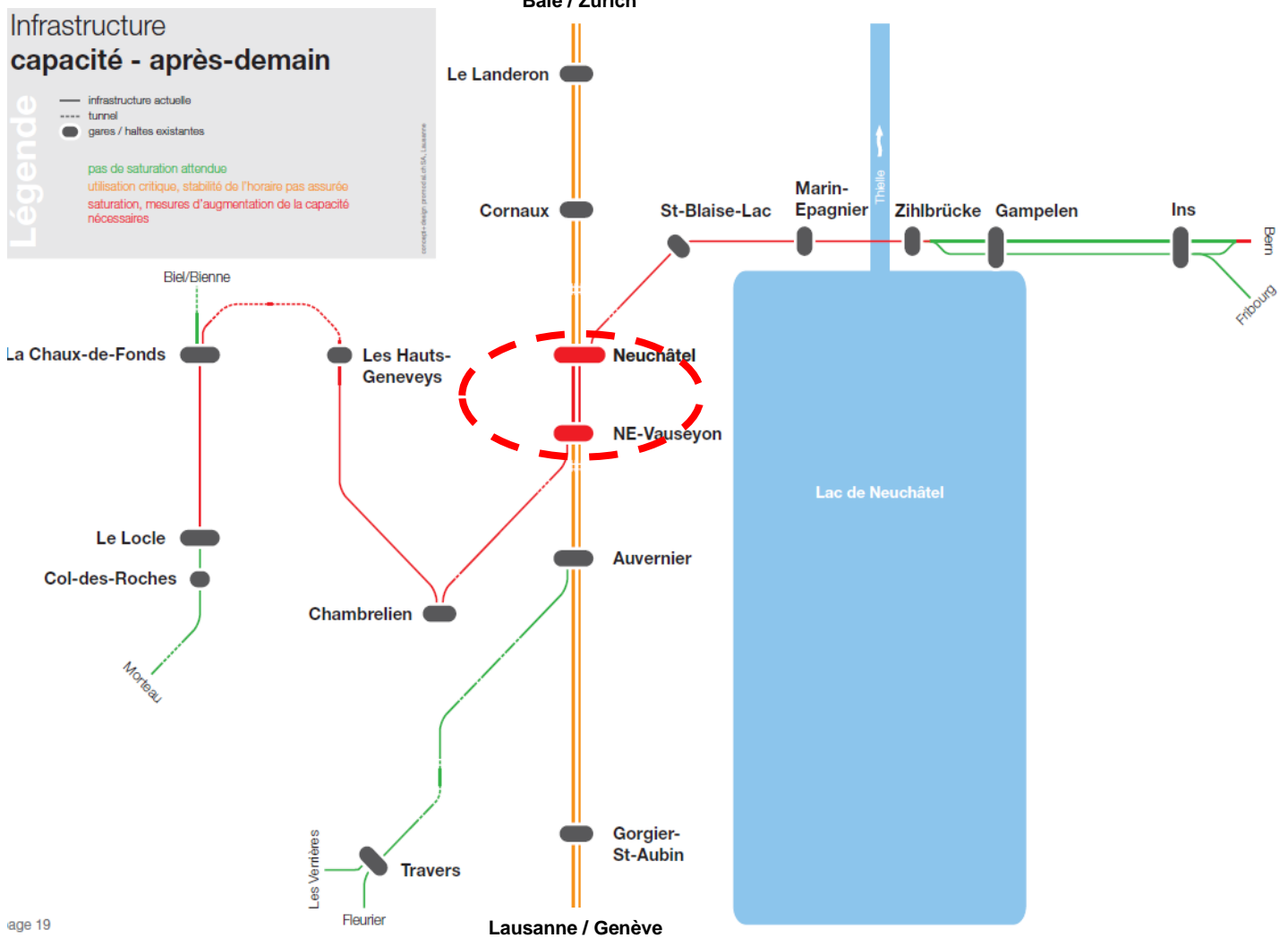
Figure 1 : Situation actuelle : Goulet d'étranglement de Vauseyon selon le plan cadre CFF
