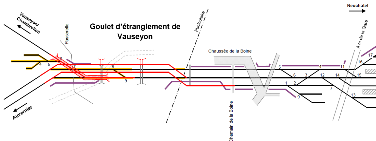
Figure 2 : 3 ème voie et désenchevêtrement pour résoudre le goulet de Vauseyon (selon étude Basler & Hofmann)
